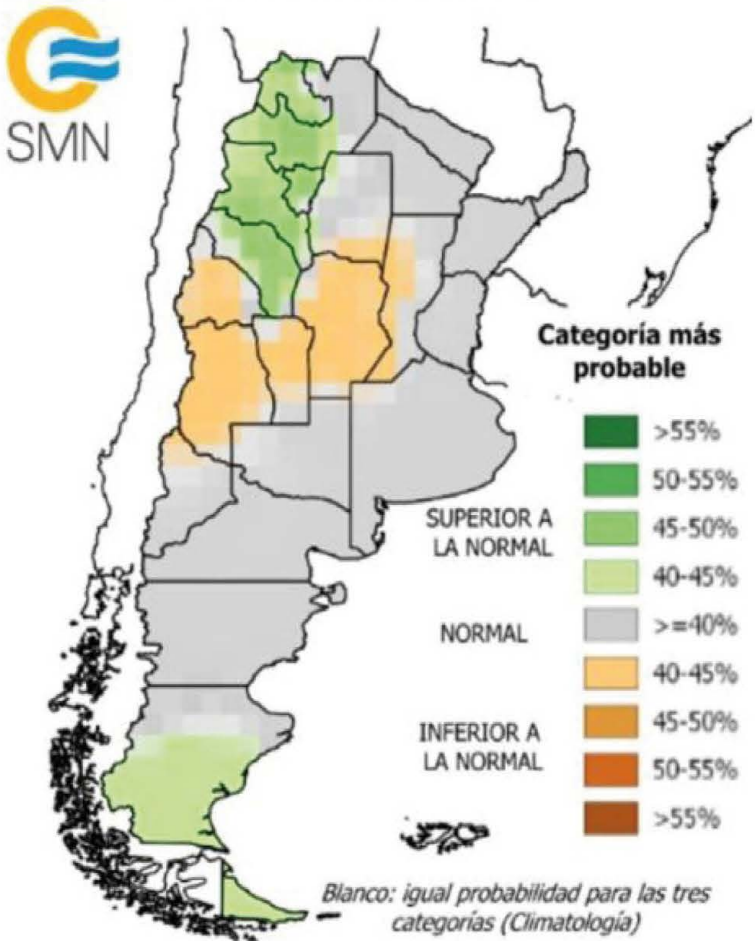
Pronóstico de Precipitación Marzo - Abril - Mayo 2026
